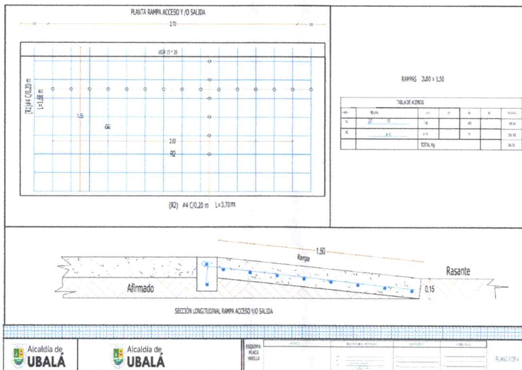
Figura 3. Detalle rampa
