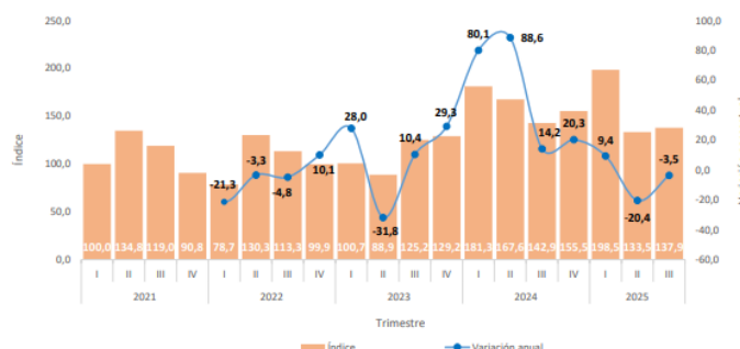
Gráfico 7. Índice y variación anual de la producción de los puentes, canales, presas, sistemas de riego y otras obras hidráulicas (acueductos) Total nacional – serie a precios constantes. 2021 (I trimestre) – 2025 (III trimestre h )
