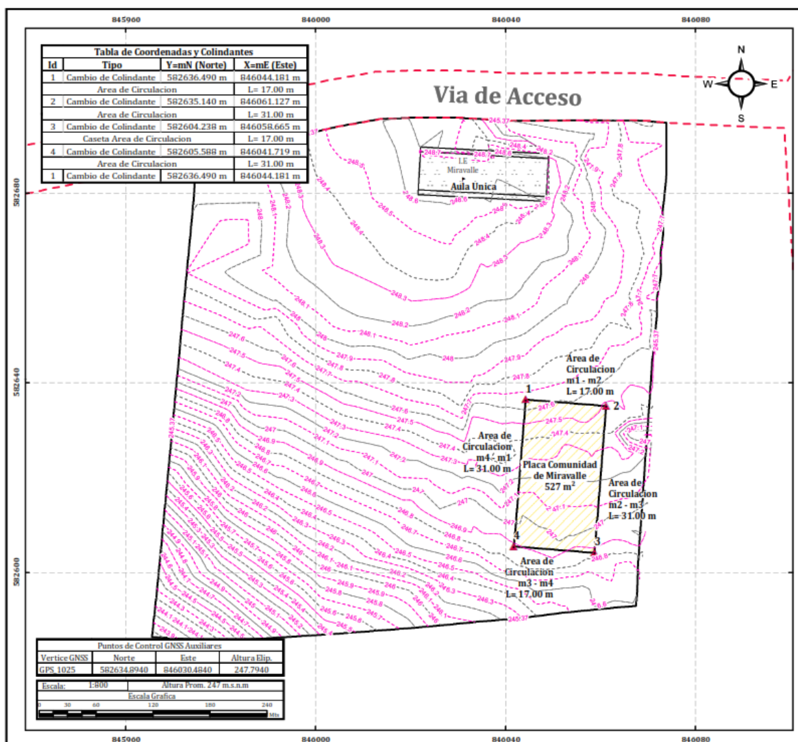
Ilustración 16. Plano de La Placa de la Institución Educativa Rural de la Vereda Miravalle
