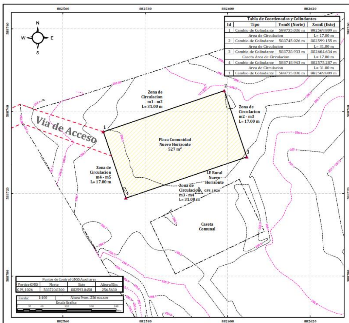
Ilustración 13. Plano de La Placa Institución Educativa Rural Nuevo Horizonte
