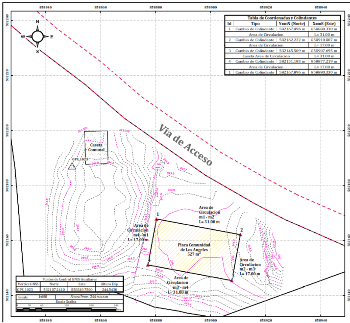
Ilustración 15. Plano de La Placa Comunidad Nuevo Amanecer
