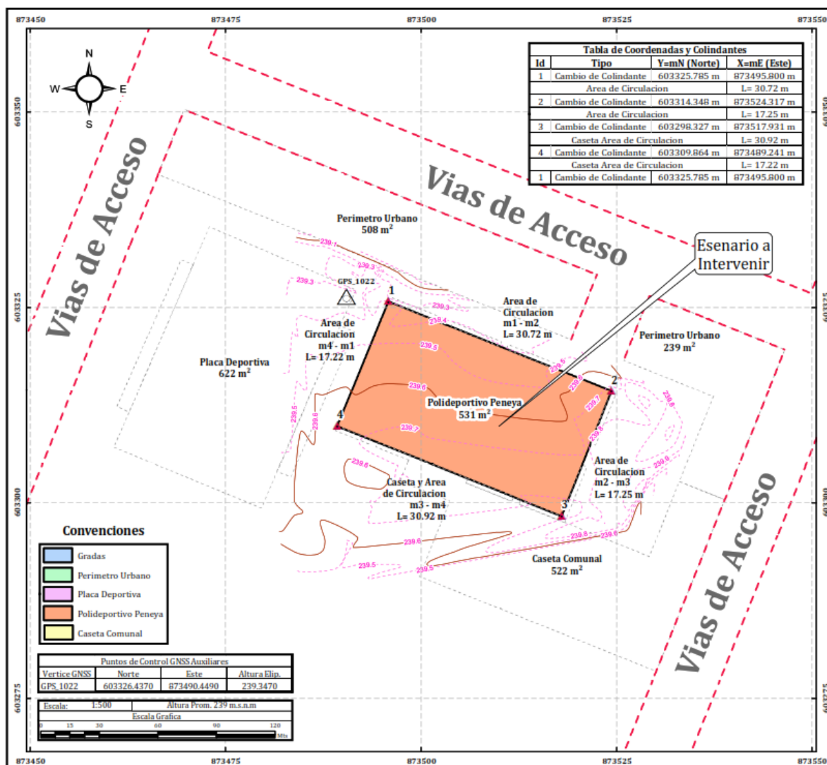
Ilustración 11. Plano del Polideportivo Campo Alegre (Peneya).
