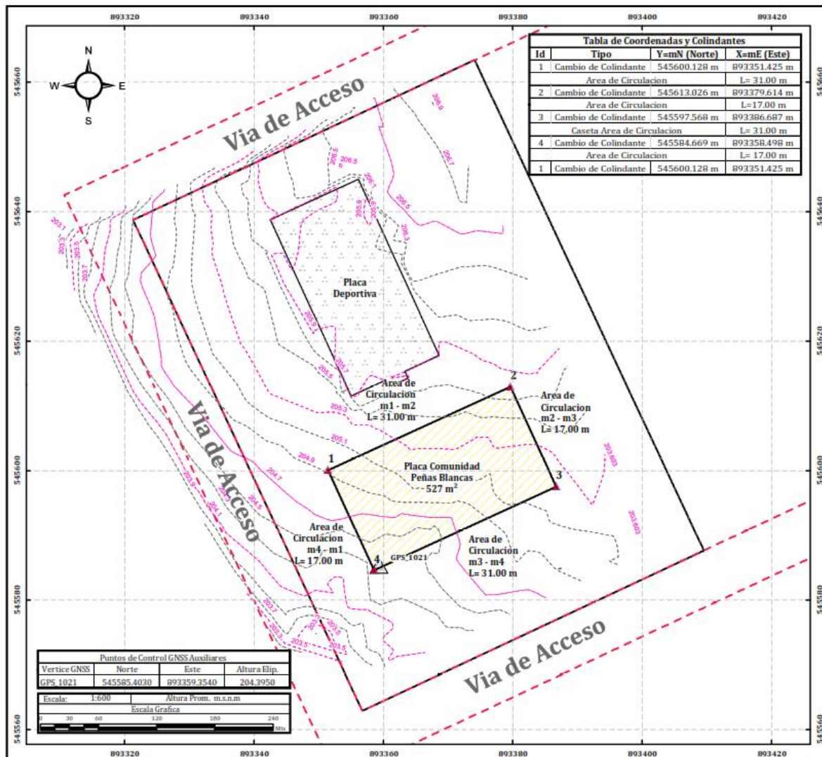
Ilustración 14. Plano de La Placa Comunidad del Centro Poblado Peñas Blancas
