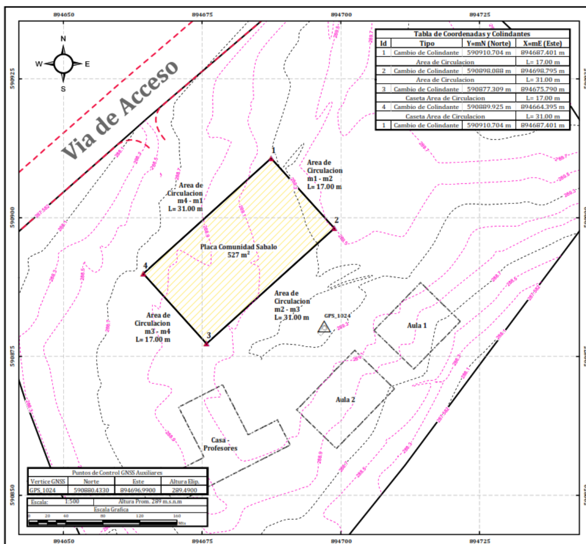
Ilustración 12. Plano de La Placa Institución Educativa Sede El Sábalo
