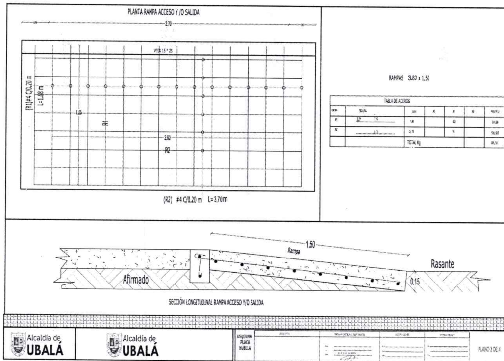
Figura 3. Detalle rampa
