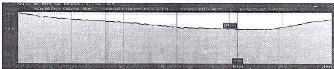
Imagen 22. Localización, registro fotográfico y perfil (mayor al 7%) Placa huella vía Inspección La Playa – Vereda Mundo Nuevo Sector La Capilla, tramo 130 metros lineales
