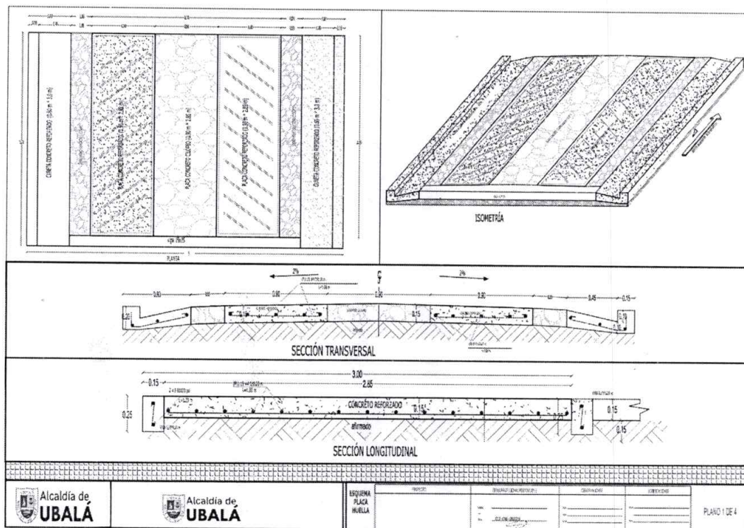
Figura 1. Secciones típicas Placa Huella
