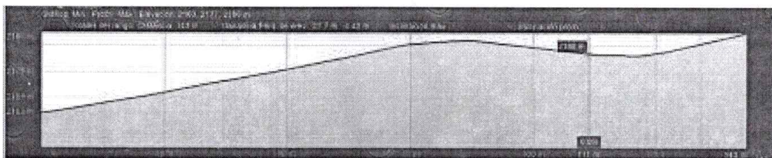
Imagen 19. Localización, registro fotográfico y perfil (mayor al 7%) Placa huella vía Vereda Santa Rosita – Inspección La Playa Sector El Pino, tramo 130 metros lineales
