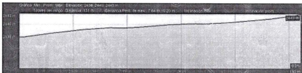
Imagen 3. Localización, registro fotográfico y perfil (mayor al 7%) Placa huella vía Vereda Laguna Azul – Vereda Sión, Sector Puente Rio Negro, tramo 130 metros lineales
