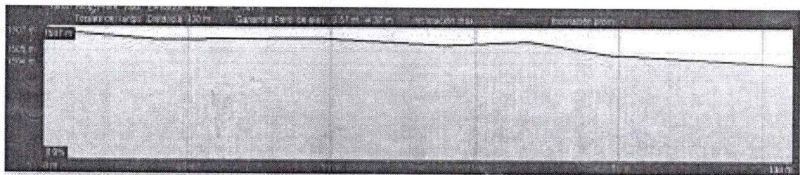
Imagen 28. Localización, registro fotográfico y perfil (mayor al 7%) Placa huella vía Inspección Santa Rosa – Vereda San Antonio Sector Pedro Díaz, tramo 130 metros lineales
