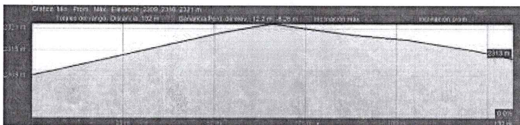
Imagen 5. Localización, registro fotográfico y perfil (mayor al 7%) Placa huella vía Vereda Laguna Azul – Vereda Sión, Sector El Colegio, tramo 130 metros lineales
