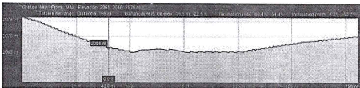
Imagen 15. Localización, registro fotográfico y perfil (mayor al 7%) Placa huella vía Vereda Santuario– Vereda Río Negro, Sector Empedrado, tramo 130 metros lineales
