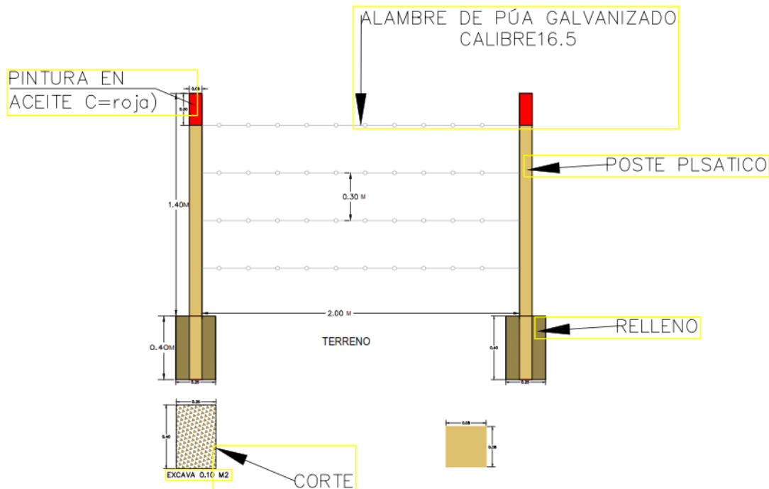
Figura 1. DETALLE AISLAMIENTO. Equipo Técnico.
