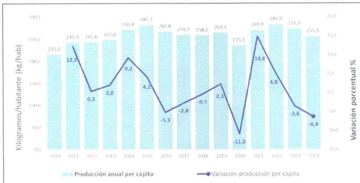
Ilustración 9. Producción anual per cápita de cemento gris 2010-2024. Fuente: DANE.
