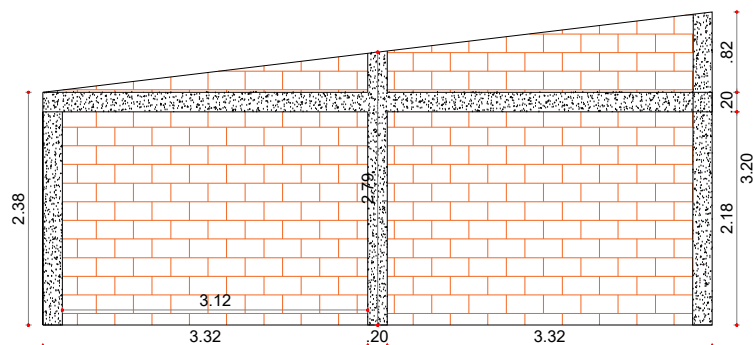
Corte 3'-3', MURO EN DIVISORIO H-10
