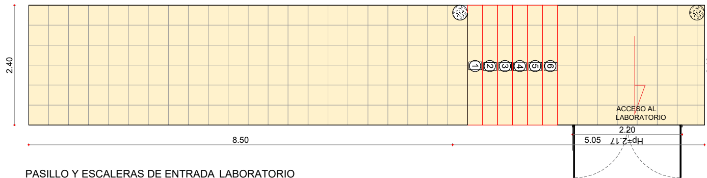
PASILLO Y ESCALERAS DE ENTRADA LABORATORIO
