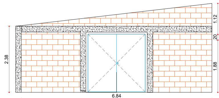
FACHADA DEL LABORATORIO
