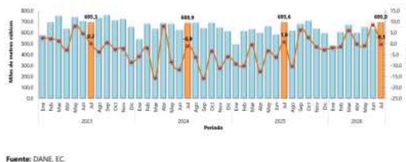
Gráfico 2. Producción de concreto premezclado (miles de metros cúbicos y variación anual) Total nacional Enero 2023 - julio 2026 P
