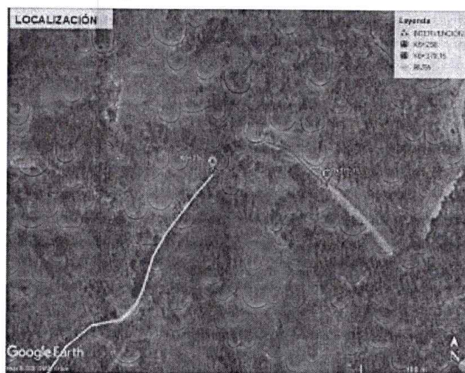
Imagen 15. Localización, registro fotográfico y perfil (mayor al 7%) Placa huella vía Vereda Santuario– Vereda Río Negro, Sector Empedrado, tramo 130 metros lineales
