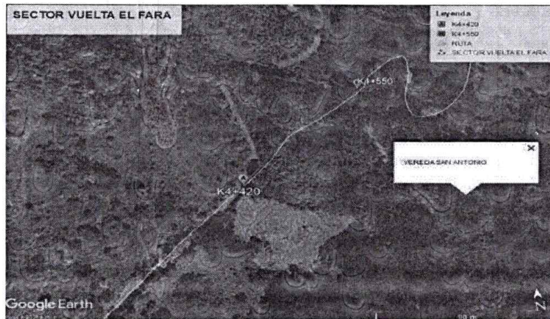
Imagen 24. Localización, registro fotográfico y perfil (mayor al 7%) Placa huella vía Vereda San Antonio – Vereda El Carmen Sector Vuelta del Fara, tramo 130 metros lineales
