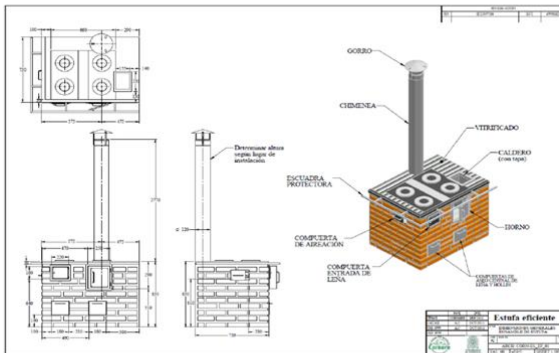
Figura 1. Diseño de la Estufa Eficiente.
